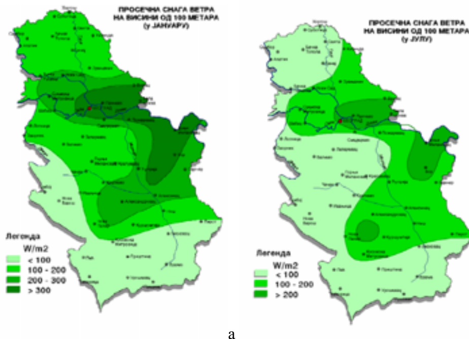
Sl. 4 Atlas vetra Srbije- Studija EE704-1052A projekat iz 2005. god. CMS /6/
