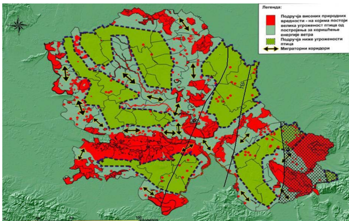
Sl. 9 Poređenje karte velike ugroženosti ptica i karte energetskog potencijala vetra
